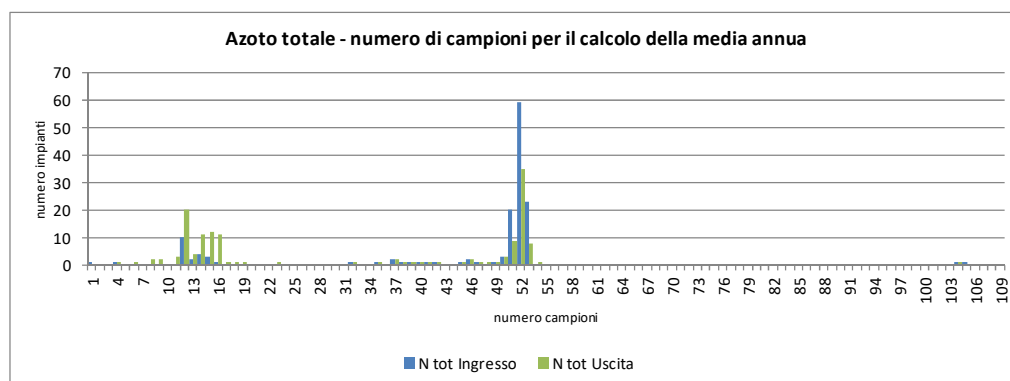
Figura 18. Distribuzione delle frequenze mensili di campionamento ed analisi, parametro Azoto totale; tutti gli impianti di potenzialità compresa tra 2.000 e 9.999 AE.
