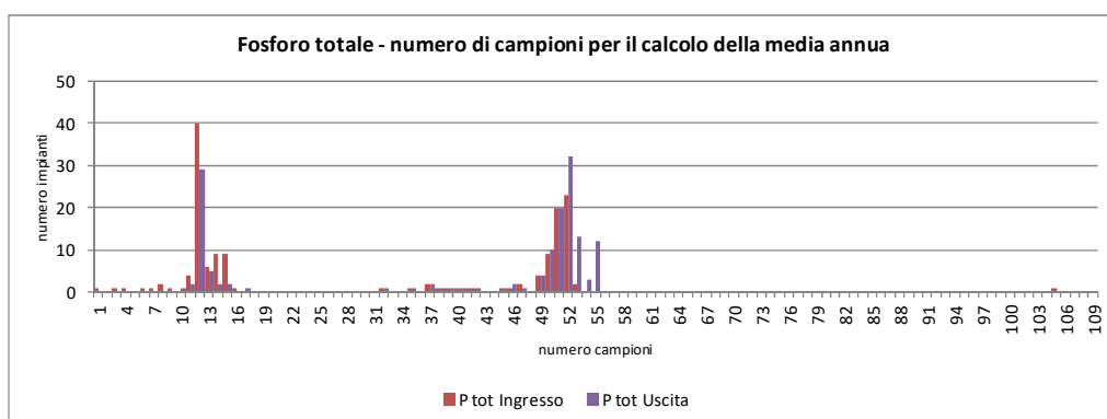
Figura 19. Distribuzione delle frequenze mensili di campionamento ed analisi, parametro Fosforo totale; tutti gli impianti di potenzialità compresa tra 2.000 e 9.999 AE.
