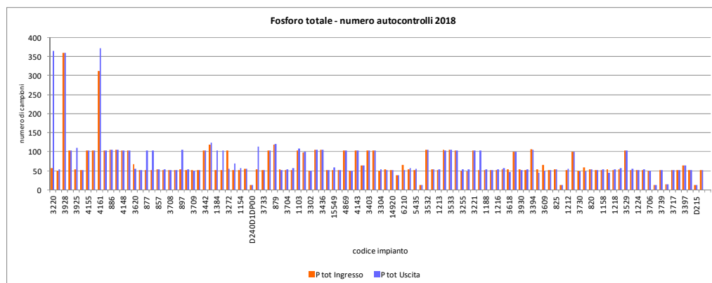
Figura 14. Numero di prelievi (ingresso e uscita) per la determinazione del Fosforo totale per singolo impianto.
