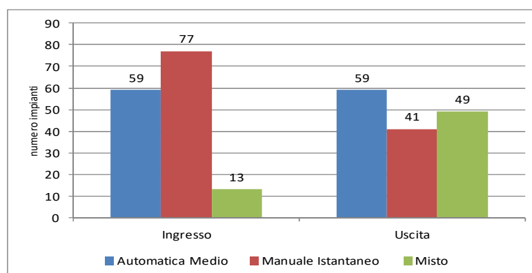
Figura 17 Metodi di campionamento adottati, per impianto.
