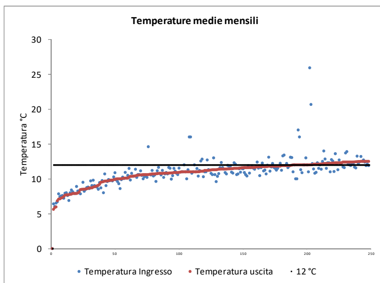
Figura 21. Particolare del grafico di Fig.20 con le temperature in ingresso e in uscita < 12^{\circ}\text{C}
